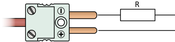
Obrázek 11.17: RTD v dvouodičovém zapojení s miniaturním konektorem
